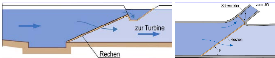
Figure 6 : plan de grille incliné par rapport au lit (à gauche) et orienté par rapport aux parois du chenal (à droite) - (Dumont et al, 2005).
